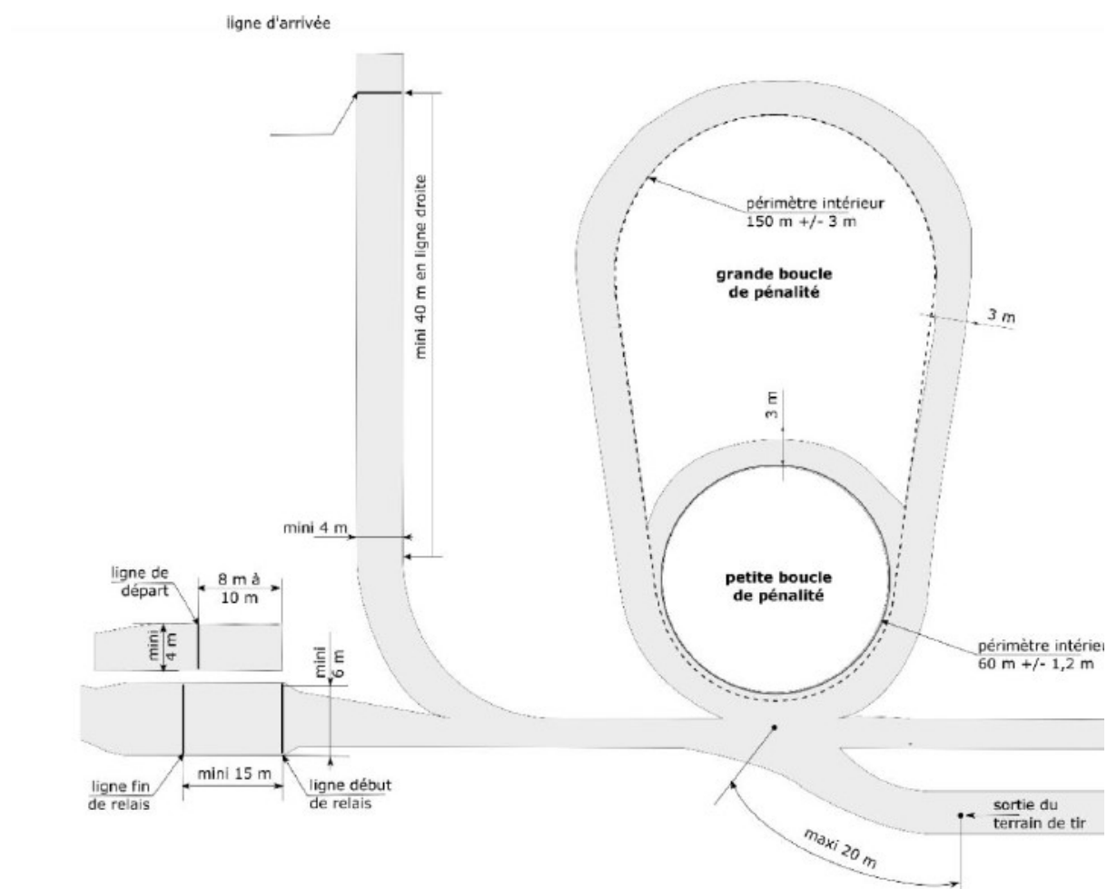
Annexe 3 : Dimensions des zones et distances
